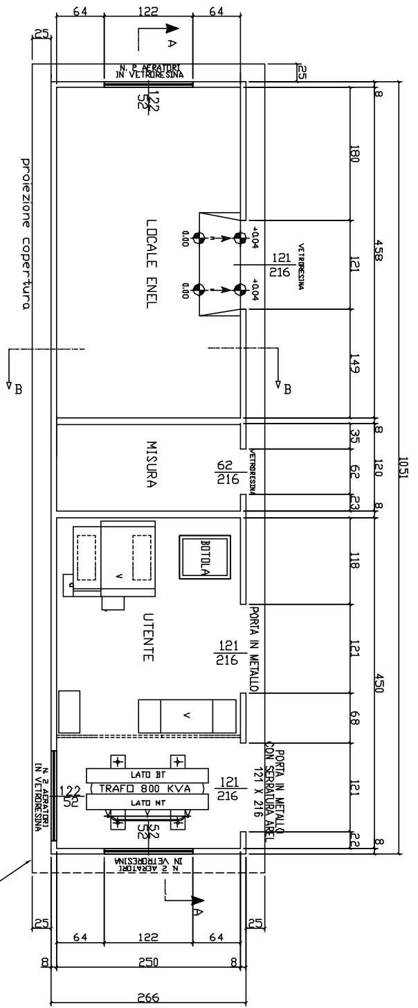
PIANTA CABINA
