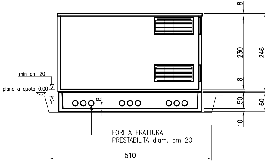
SEZIONE A-A
