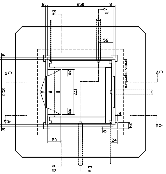
PIANTA DELLA CABINA
