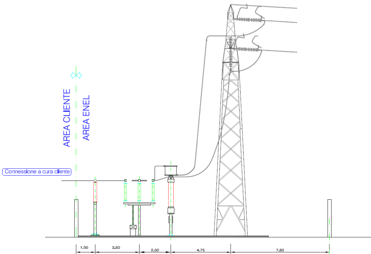
Figura E-4: Vista impianto di rete per la consegna in antenna o derivazione rigida a "T"
