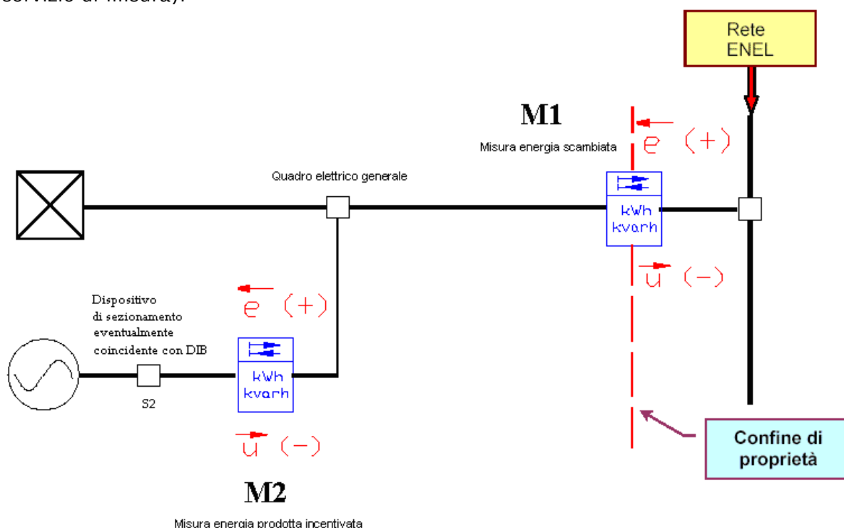
Figura H-1 Schema di collegamento dei sistemi di misura Enel presso un Produttore con servizio di scambio sul posto o che effettua la cessione “parziale” in rete dell'energia prodotta.
