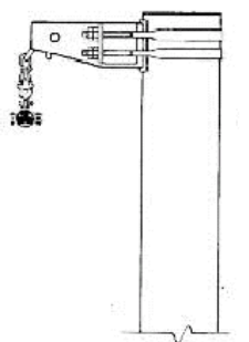
Mensola per cavo aereo
