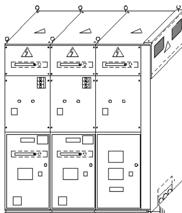
Figura G-15: Scomparti MT con isolamento misto (a) e in aria (b)
